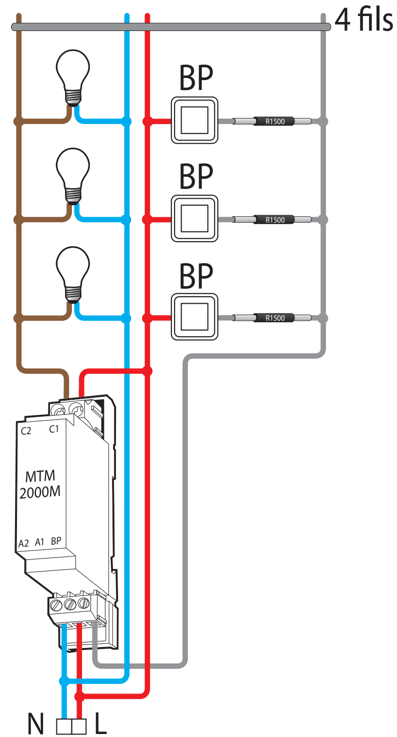
Câblage MTM2000M avec R1500 antiblocage - commun à la phase
