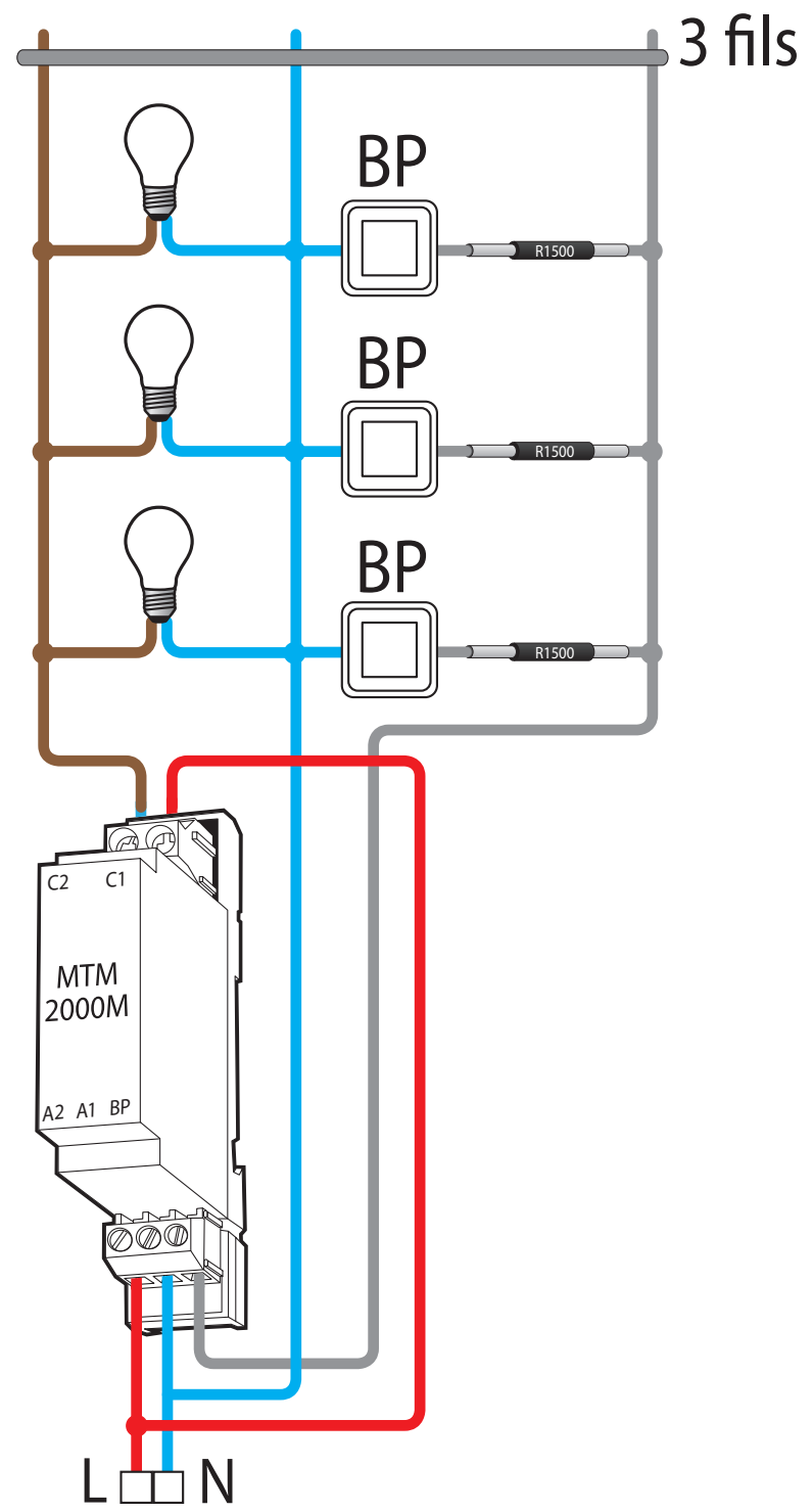
Câblage MTM2000M avec R1500 antiblocage - commun au neutre
