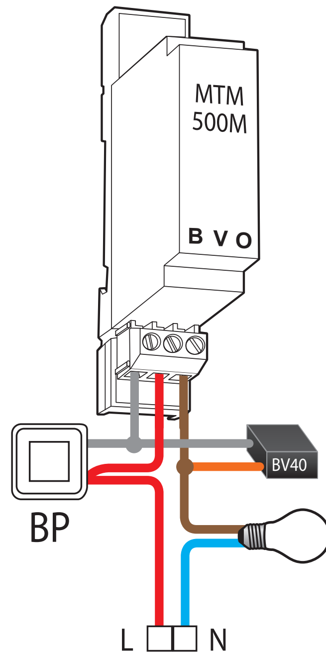
Câblage MTM500M avec BV40 - commun à la phase
