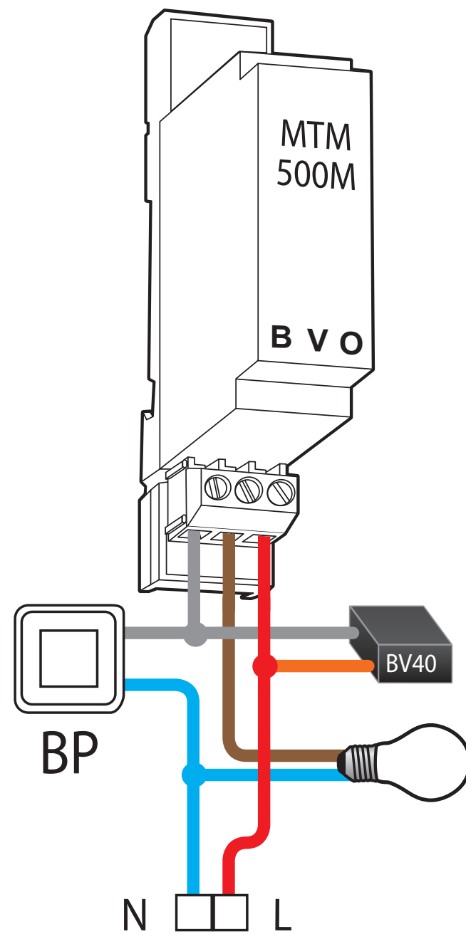
Câblage MTM500M avec BV40 - commun au neutre
