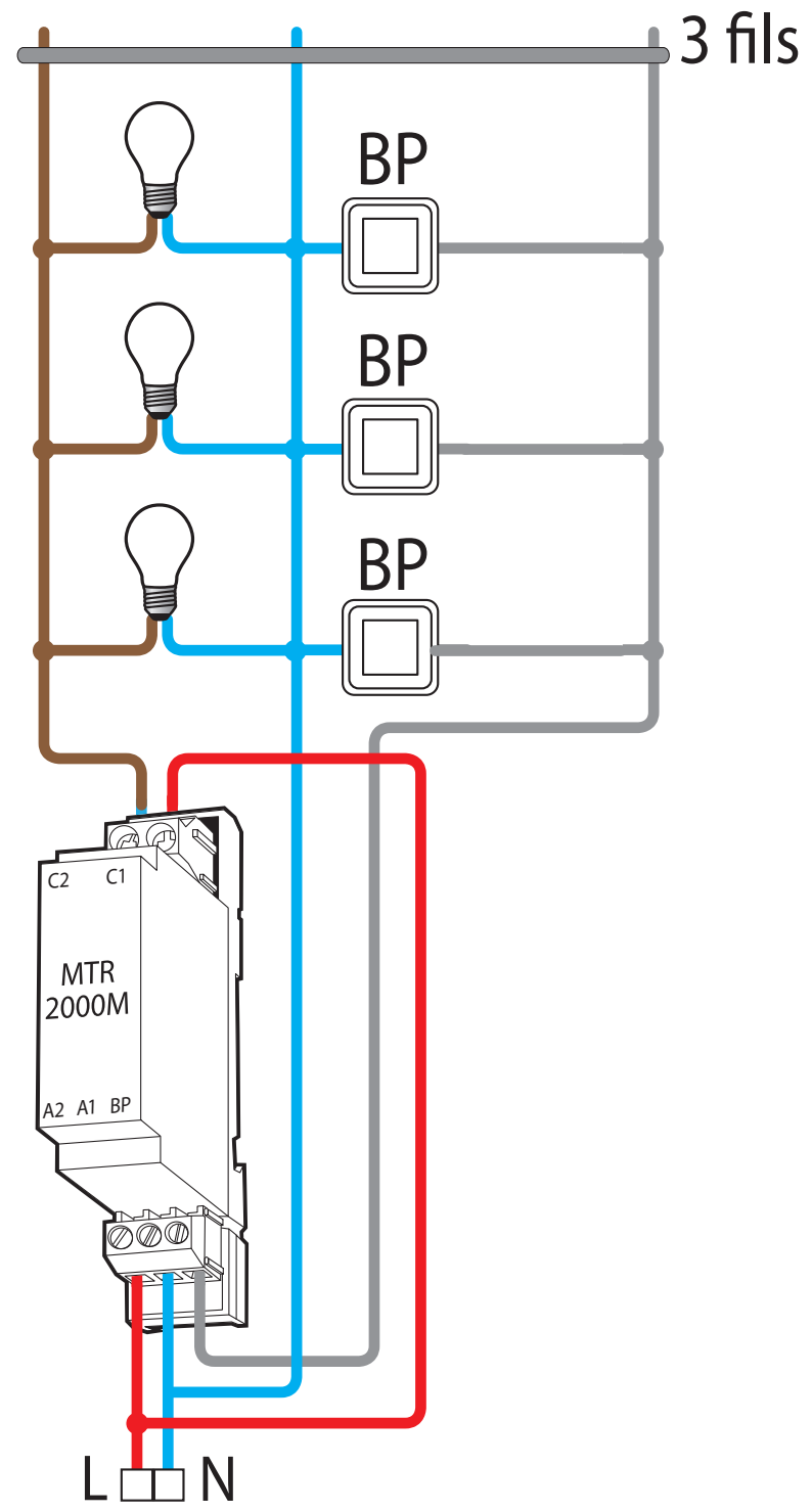
Câblage MTR2000M - commun au neutre
