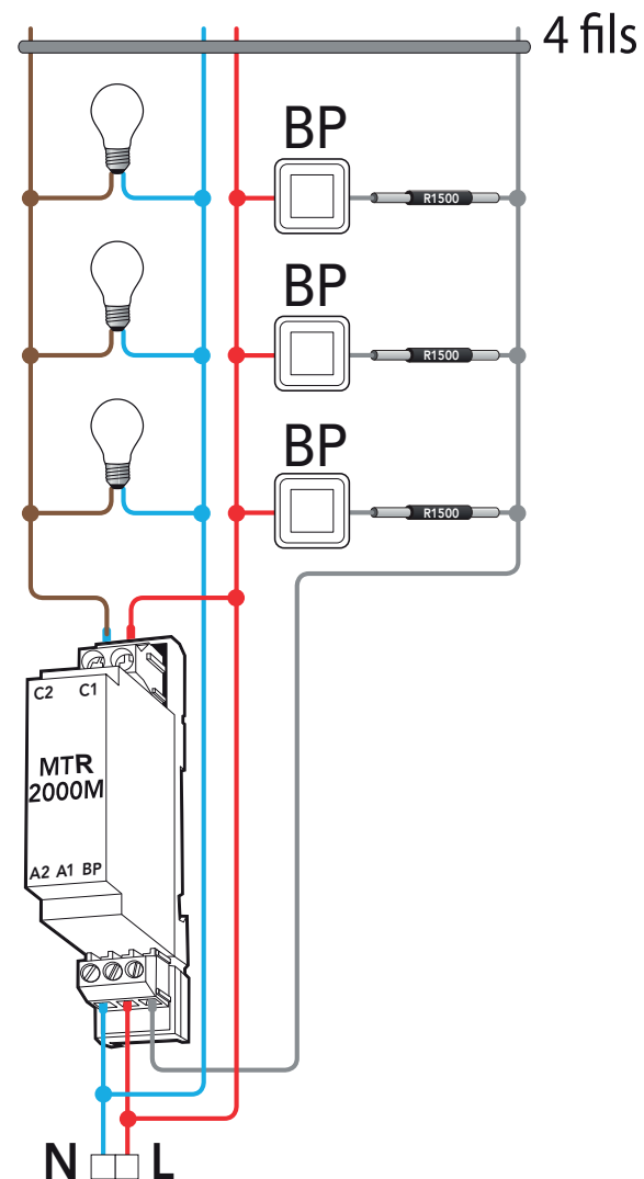
CABLAGÉ AVEC LE COMMUN DES POUSOIRS A LA PHASE
