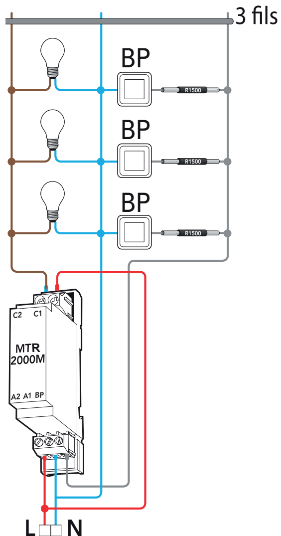
CABLAGÉ AVEC LE COMMUN DES POUSOIRS AU NEUTRE
